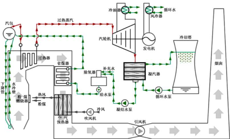
火力发电流程
