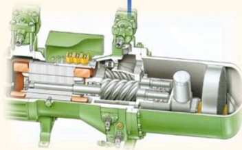
压缩机
