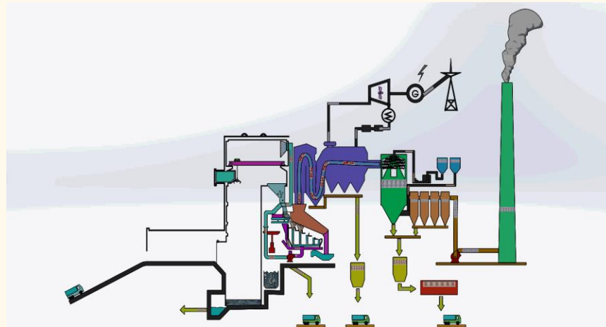
垃圾发电流程
