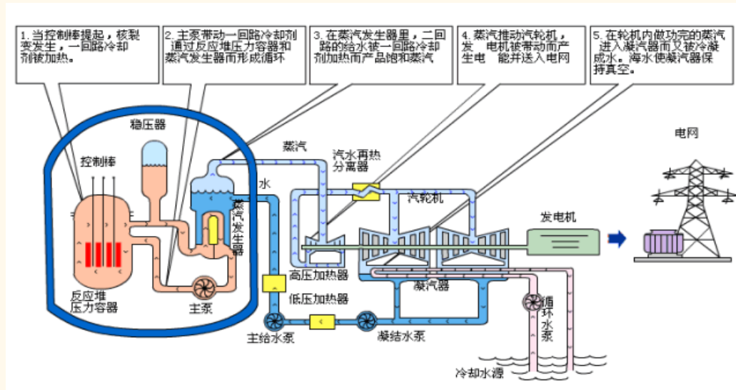
核能发电流程
